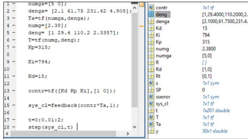
Fig. 5: The PID controller parameters
