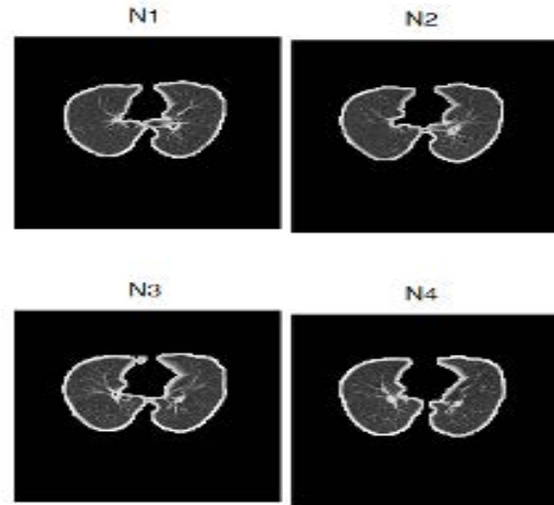
Fig. 4: Output images
